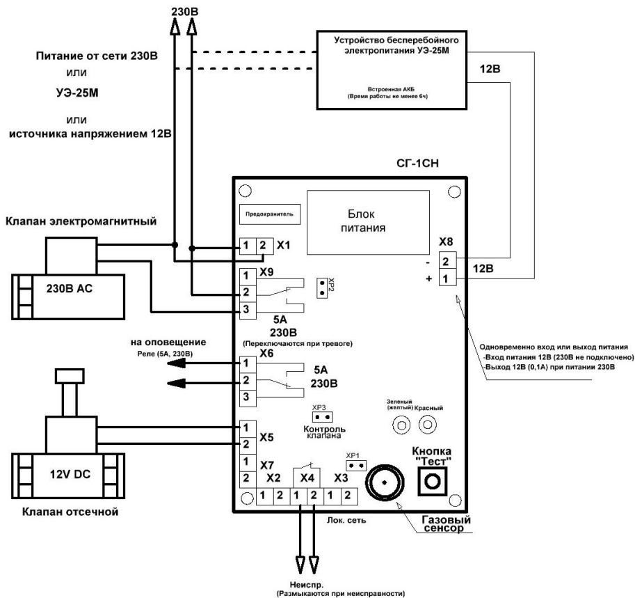
Схема подключения сигнализатора от источника бесперебойного питания УЭ-25М Рис. 8
